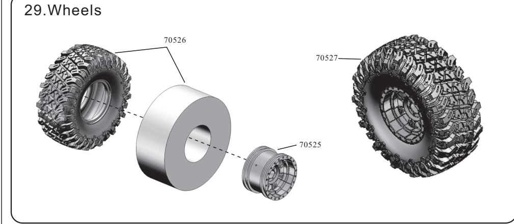
29. Wheels
