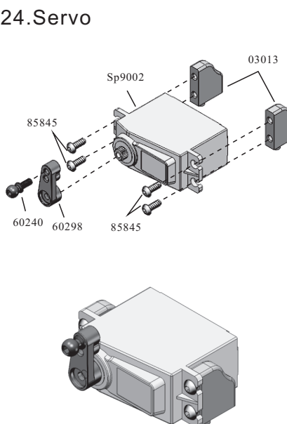
24. Servo
