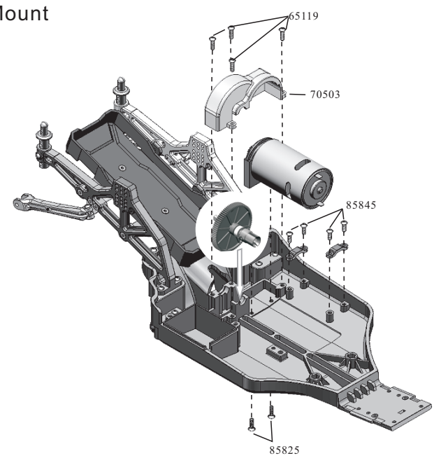
21. Motor Mount
